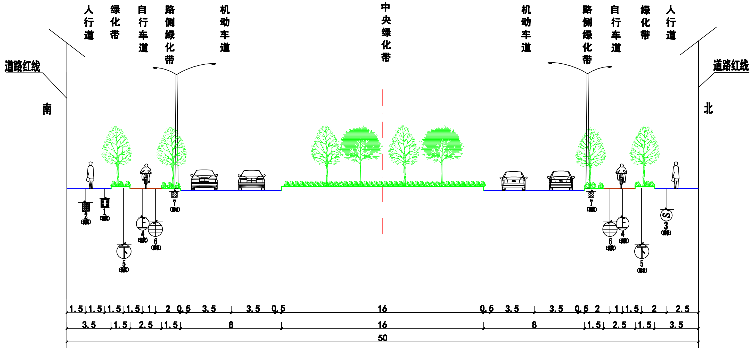
鹿角园路(云树路-龙洲路)规划横断面
