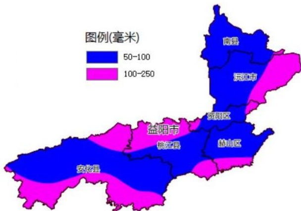
图 1 18 日晚~21 日白天累积降水量预报
